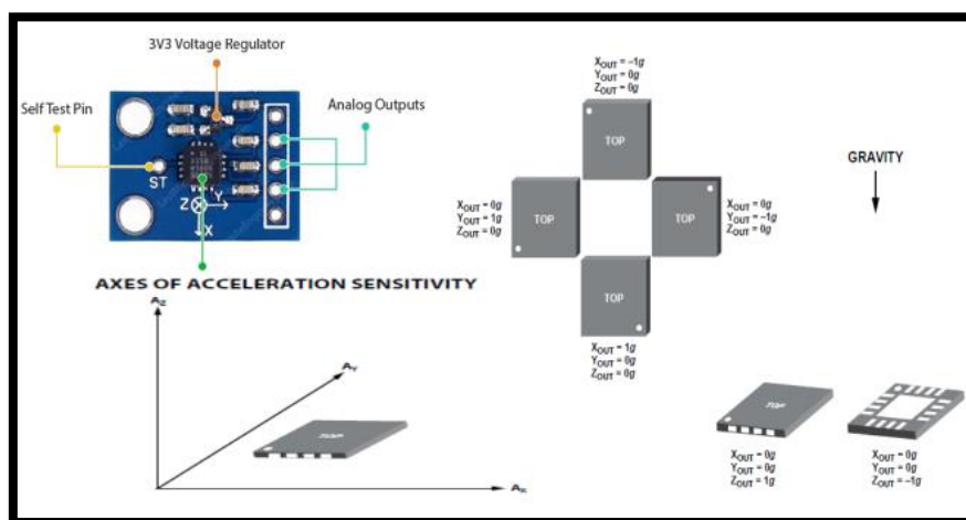
Fig.4. MEMS Accelerometer module
